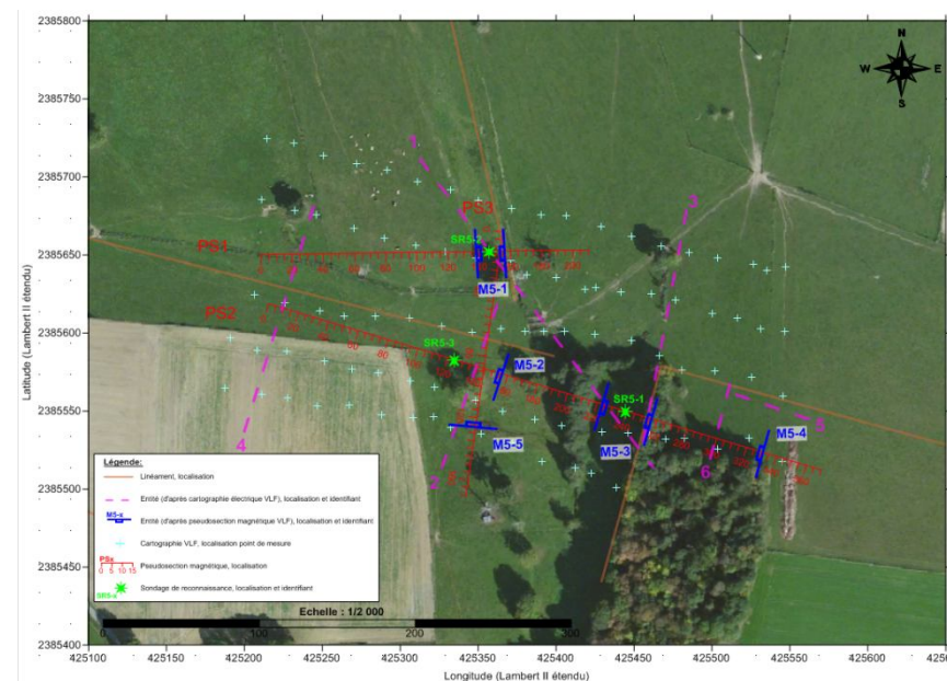
Synthèse des résultats d'une prospection VLF - Implantation des sondages de reconnaissance (Calligée)
