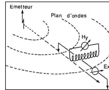
Propagation des ondes électromagnétiques (Grissemann et Reitmayr)
