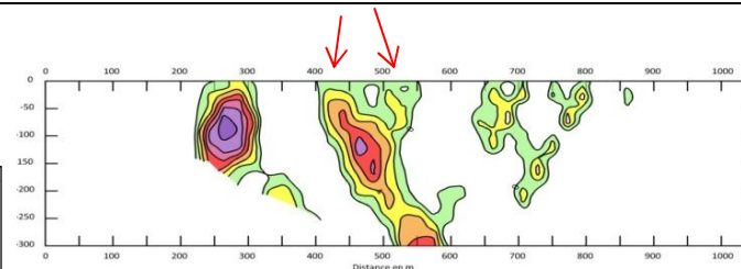
Grand-Champ (Morbihan) - Représentation de la pseudosection magnétique en travers des structures décrites plus haut
