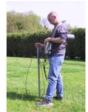
Résistivimètre de type IGS-2/VLF-4 construit par Scintrex (Calligée)
