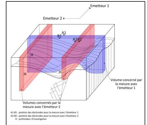
Représentation de l'effet directionnel des mesures (Calligée)
