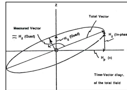
Ellipse de polarisation du champ magnétique au droit d'un conducteur (Geonics)
