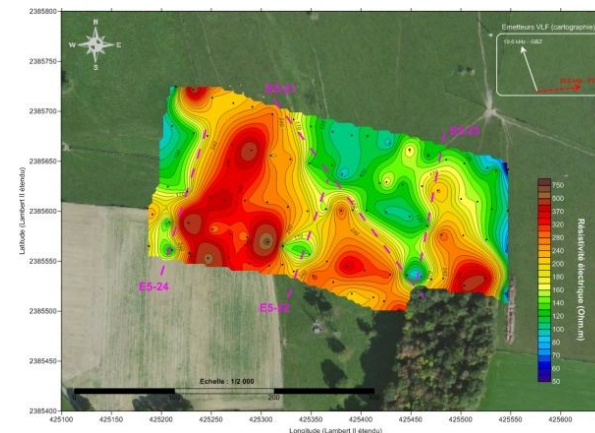
Cartographie de résistivités apparentes (Calligée)
