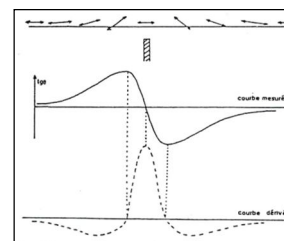
Représentation des variations de l'angle d'inclinaison du champ magnétique
