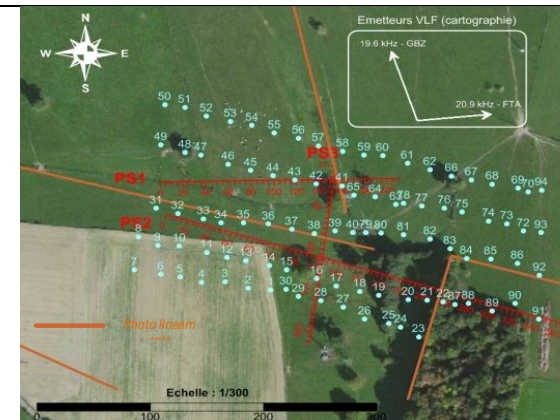
Implantation des points de mesures maille 20 x 40 m pour les résistivités (en bleu) et 5 m pour les pseudosections (en rouge) réalisées après la réalisation des cartes de résistivités (Calligée)
